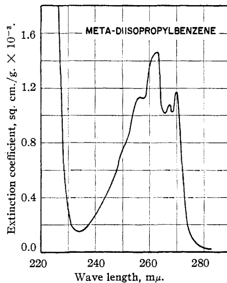
Fig. 4.—Ultraviolet spectrum of m -diisopropylbenzene.
