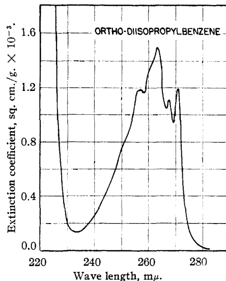
Fig. 3.—Ultraviolet spectrum of o -diisopropylbenzene.
